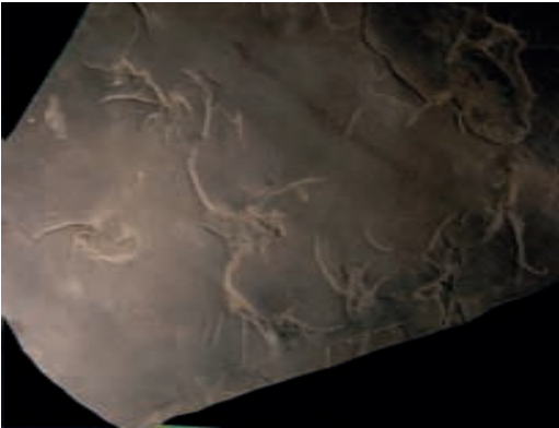
Dromopus didactylus
